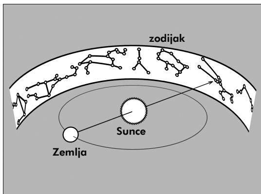
Slika 2: Kako se određuje znak Zodijaka
