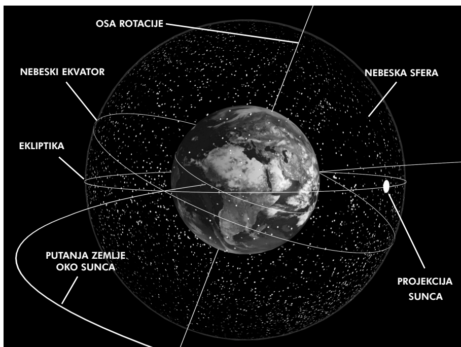
Slika 1: Zemlja i nebeska sfera
