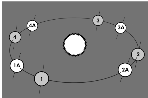
Slika 4: Pomeranje tačke ravnodnevnice
