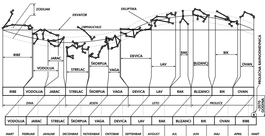
Slika 5: Pomeranje znakova zodijska usled precesije
